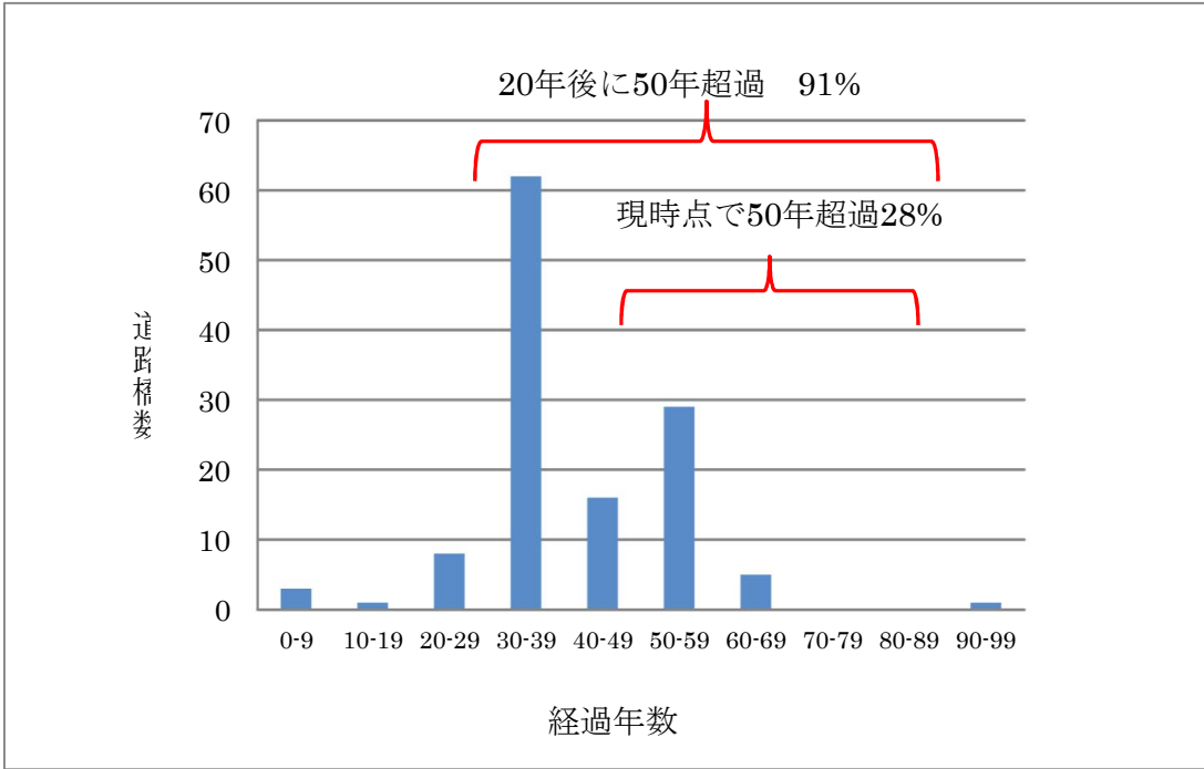
図 2 - 1 川本町が管理する道路橋の経過年数ごとの橋梁数
